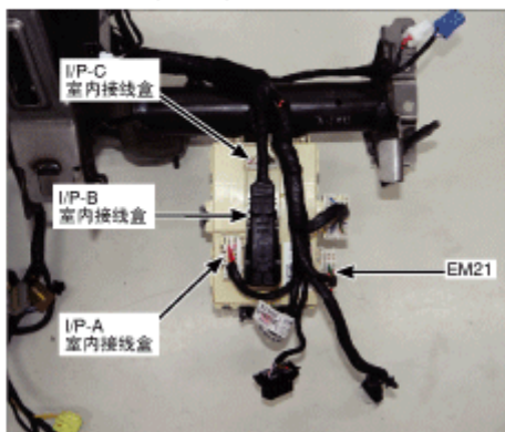
32. 仪表板左侧(后视图)
