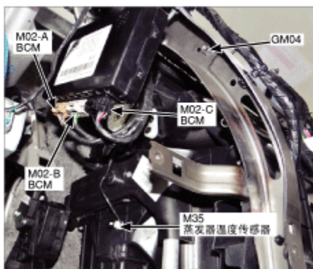
35. HVAC壳体左侧
